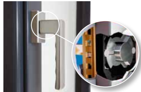
POIGNÉE AVEC SYSTÈME SECUSTICK® REND IMPOSSIBLE L'OUVERTURE DU MÉCANISME PAR L'EXTÉRIEUR
