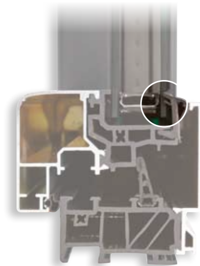
VITRAGE COLLÉ CE PROCÉDÉ DE FABRICATION REND L'ACCÈS PAR L'EXTÉRIEUR TRÈS DIFFICILE EN CAS DE TENTATIVE D'INTRUSION
